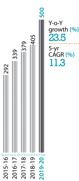
EBITDA (₹ crore)
